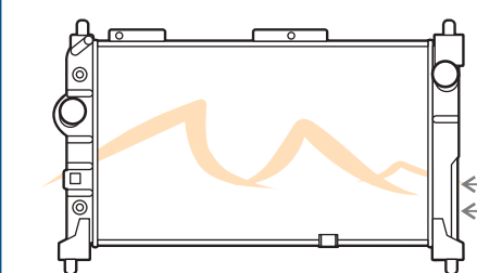
Sin sensores
